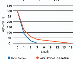
HYDRO CYCLONIC vs SKIM FILTRATION Test zmętnienia z użyciem 2,5 kg pyłu
