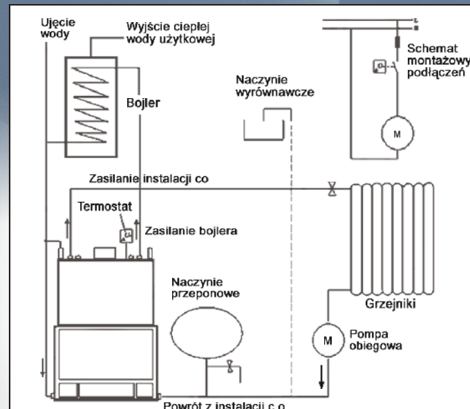
TAPIS HYDRO - urządzenie zasilające instalację centralnego ogrzewania oraz ciepłej wody użytkowej
